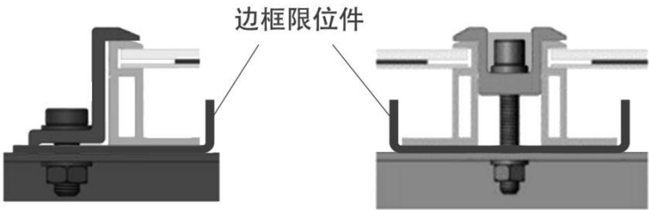
图4：边框限位件安装示意图
