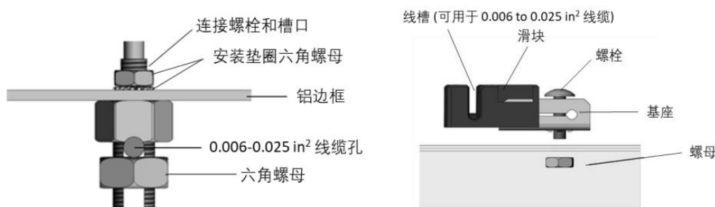
图5 光伏组件接地方法（适用于IEC）
