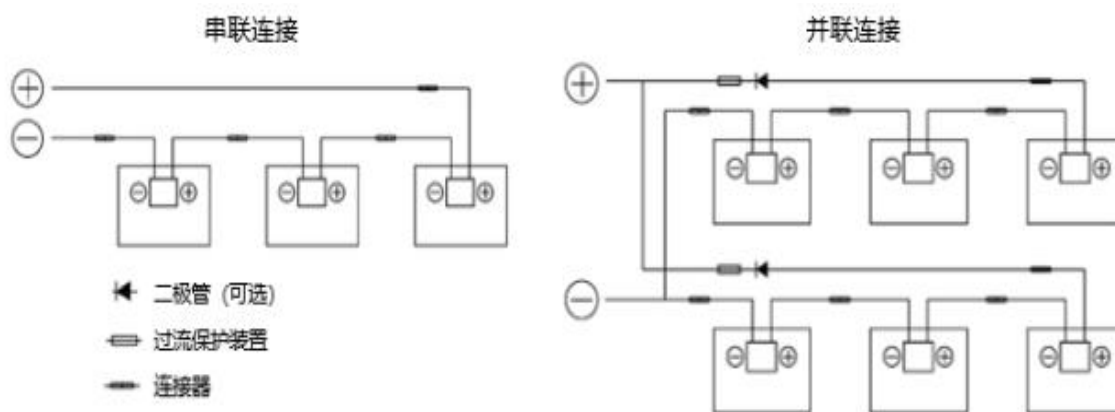
图7 串联连接和并联连接
