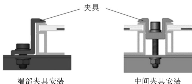
图2：普通夹具安装示意图
