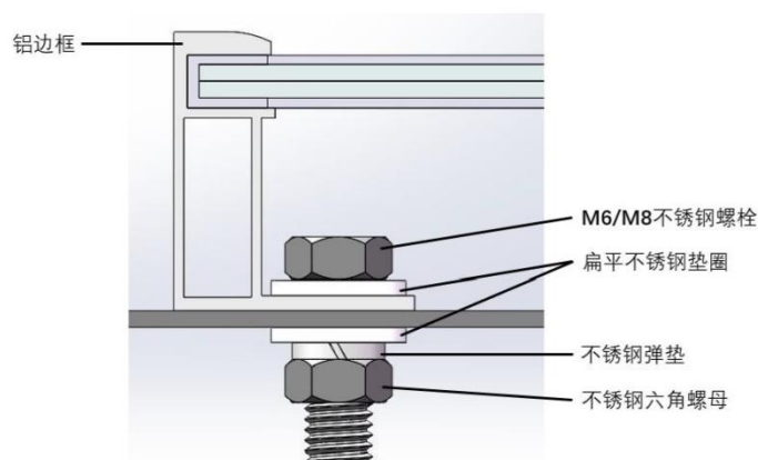
图1：使用螺栓嵌入法安装的光伏组件
