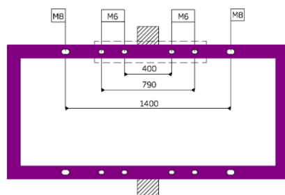
短辺に対し直角沿いのトルクチューブ 固定穴距離 400 mm/790 mm/1400 mm
