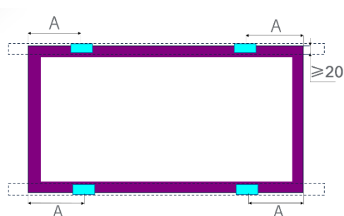
長辺 4 点クランプ固定 長辺に沿って走る架台レールに固定 レールと長辺フレームの重ね幅が 20 mm 以上あること
